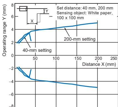
E3Z-LS@1/LS@6 BGS
