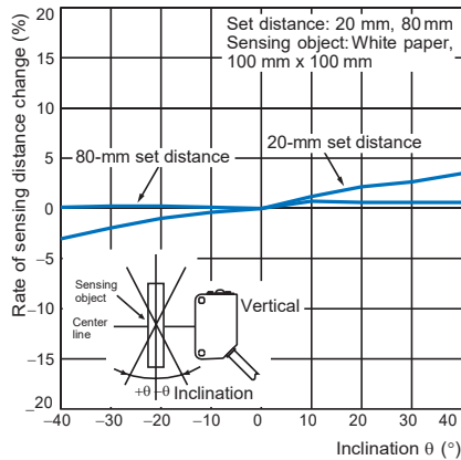
E3Z-LS@3/LS@8
