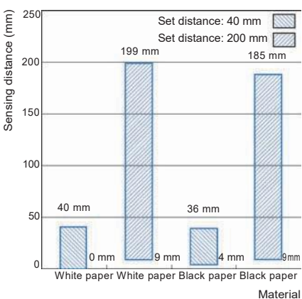
E3Z-LS@1/LS@6
