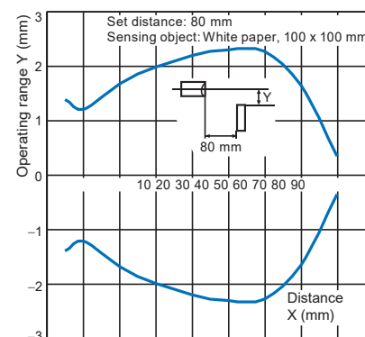
E3Z-LS@3/LS@8
