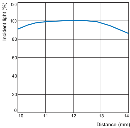
E3ZM-V@@
