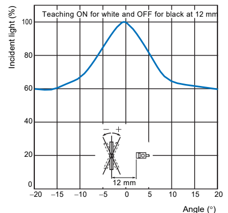
E3ZM-V@@
